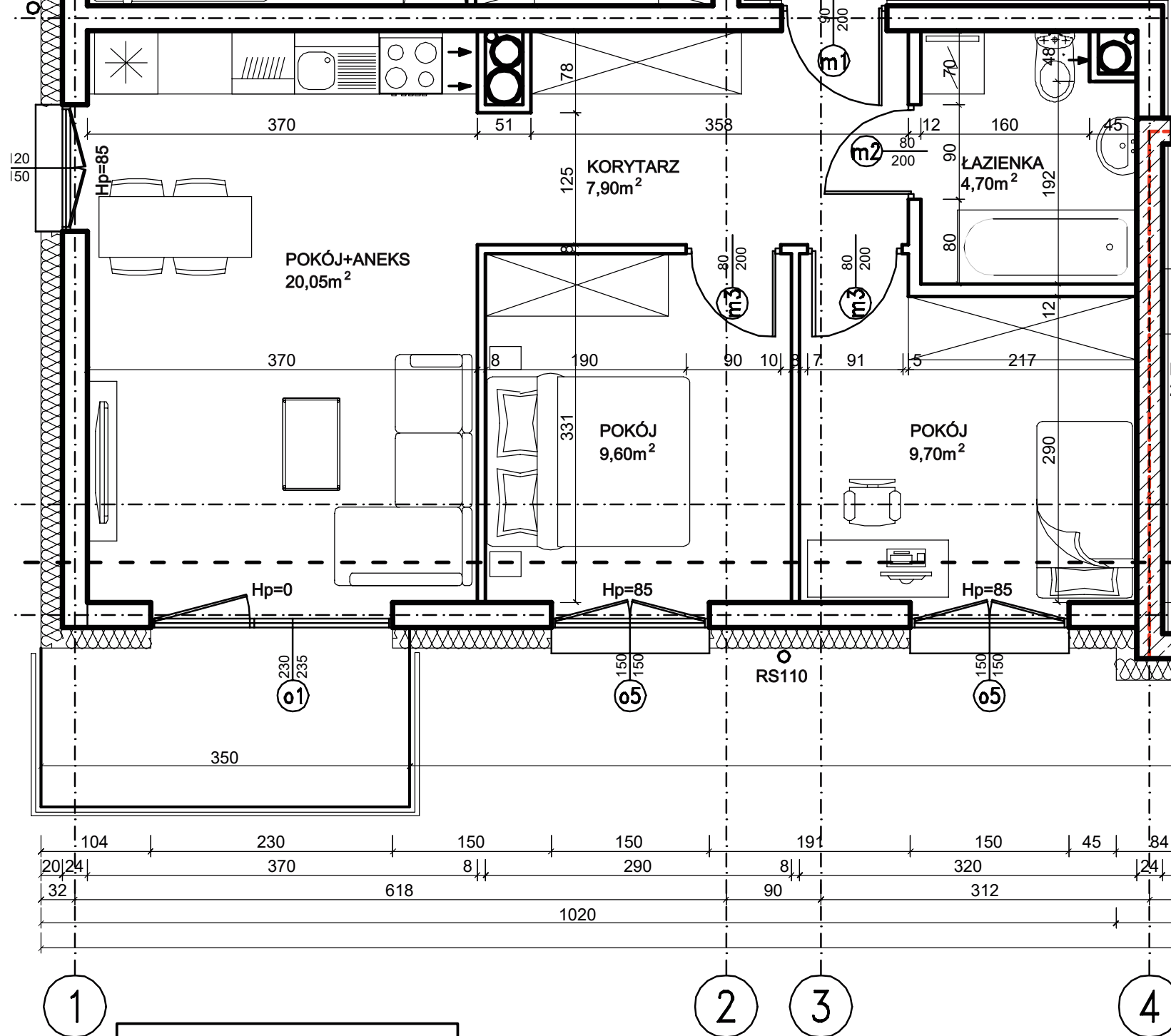
MIESZKANIE nr 92 51,95m 2
