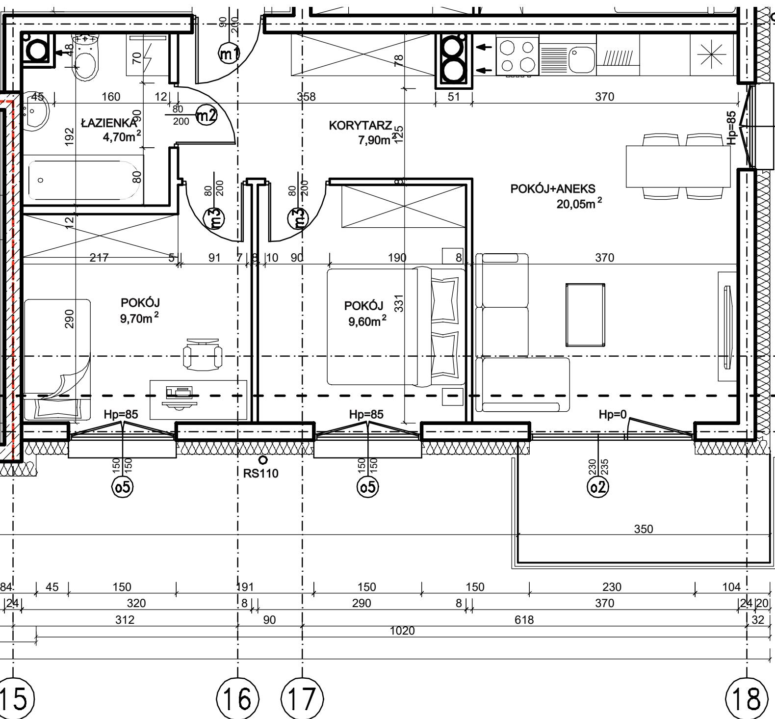
MIESZKANIE nr 35 51,95m 2
