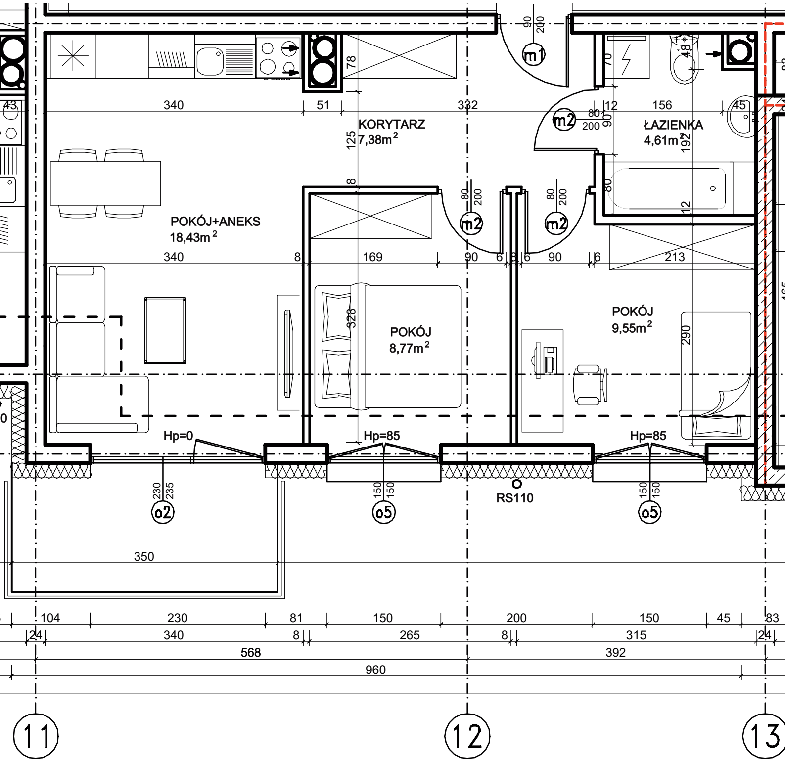
MIESZKANIE nr 29 48,74m 2
