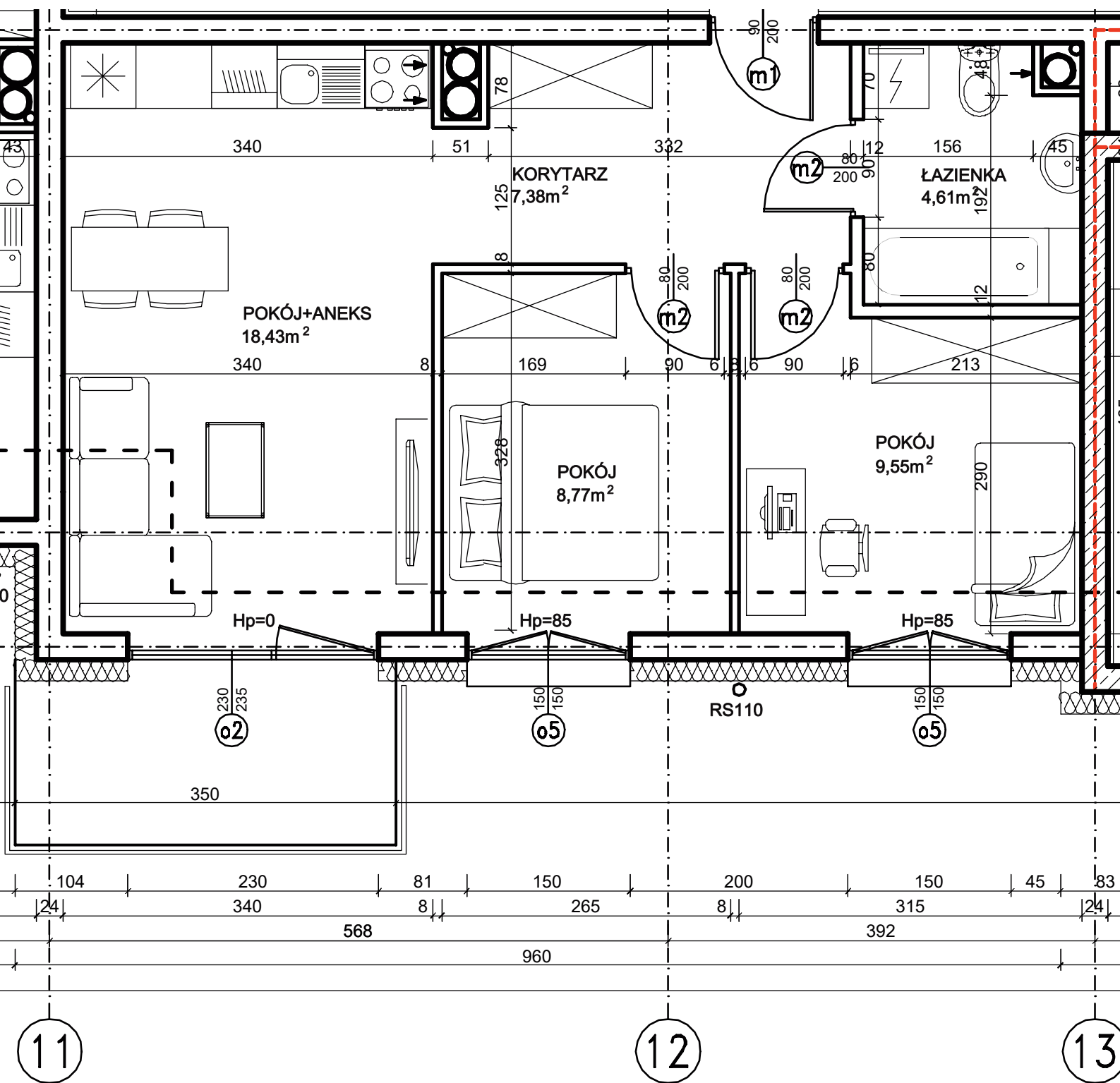
MIESZKANIE nr 15 48,74m 2
